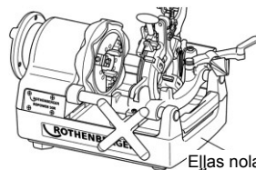
Eļļas nolaišanas skrūve
